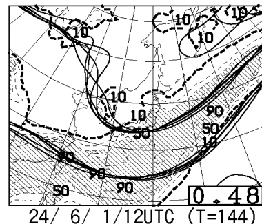
500hPa特定高度線, 降水量予想頻度分布(%)及びスプレッド
