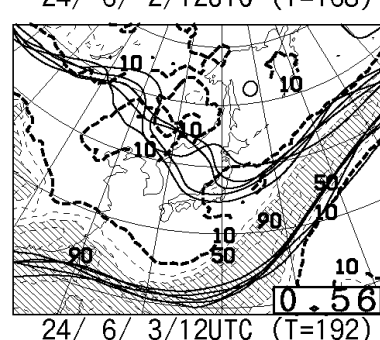
850hPaにおける気温偏差予想 (クラスター平均) 縦太線は80%, 縦細線は全メンバーの範囲
